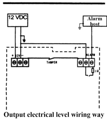
Wiring way
