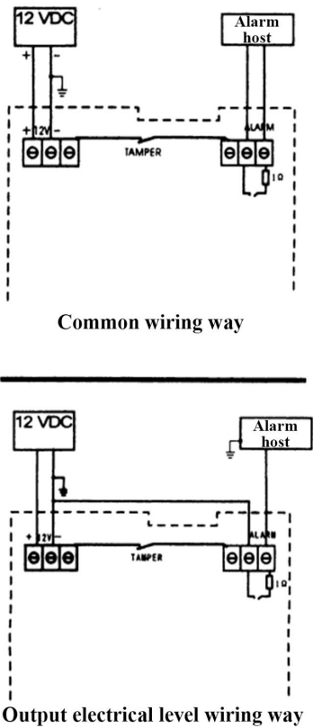
Wiring way
